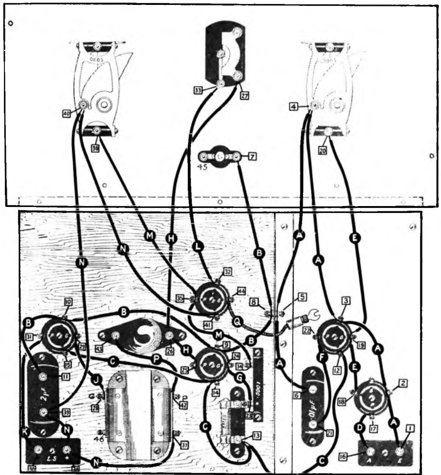
DE BOUWTEKENING DER LISSEN AFGESCHERMDE 3
