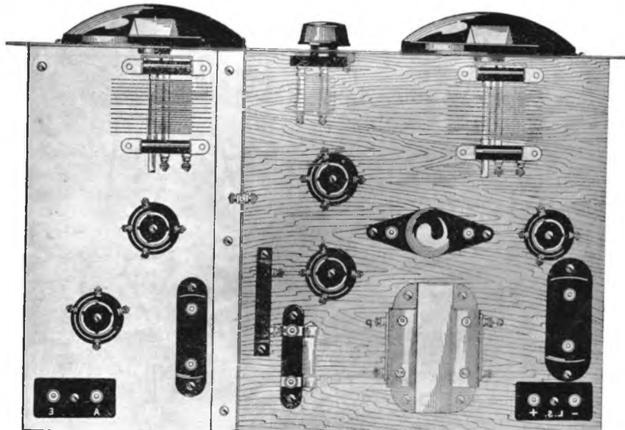
DE OPSTELLING DER ONDERDEELEN IN DEN „ONTVANGER VOOR DE FAMILIE“
